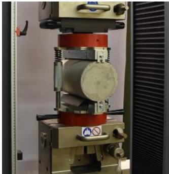
Dispositif pour essais de fendage de cylindre en béton (essai brésilien) type SPV 200
