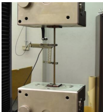
Extensomètre MFA 25
