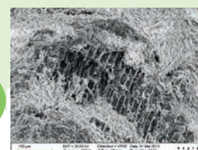
Fig. 8 : Image MEB. Biochar dans un sol maraîchier à Cocagne
