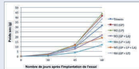
Graphique 2 Evolution de la biomasse sèche des Monocotylédones
