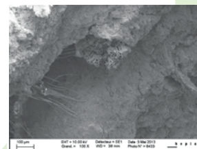
Fig. 7 : Image MEB. Biochar dans un sol maraîchier à Ayent
