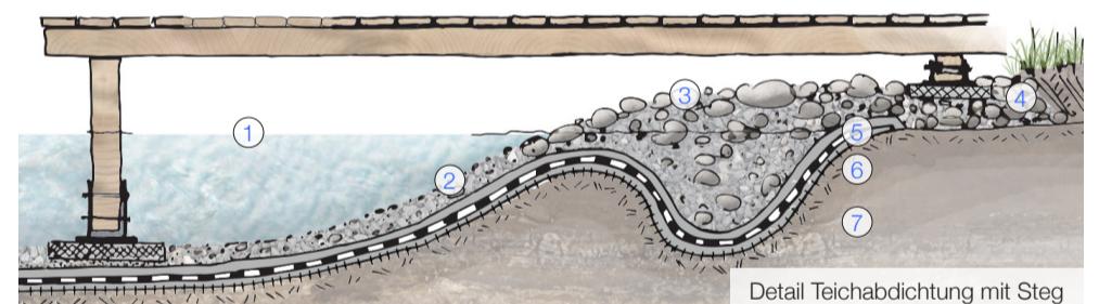
Detail Teichabdichtung mit Steg
