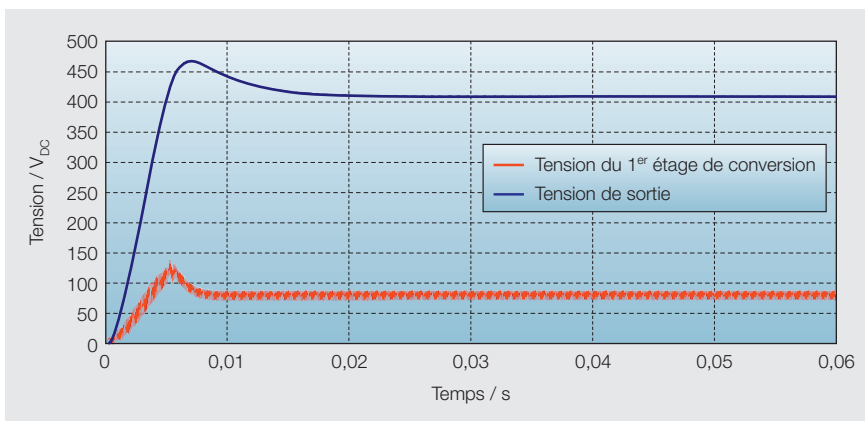
Figure 6 Résultats de la simulation du prototype de hacheur élévateur de tension (400 V DC ). En bleu la tension de sortie (aux bornes de C 2 ) et en rouge la tension du circuit intermédiaire (aux bornes de C 1 ).
