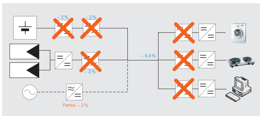
Figure 3 Schéma électrique mettant en évidence les pertes évitées (en bleu) et celles apparaissant (en rouge), telles que calculées en passant d'un environnement AC à un environnement DC.
