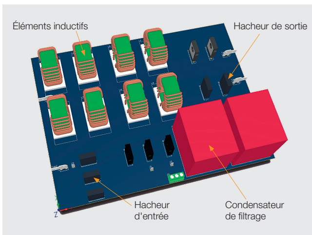
Figure 7 Prototype d'un hacheur élévateur de tension d'une puissance nominale de 1 kVA.
