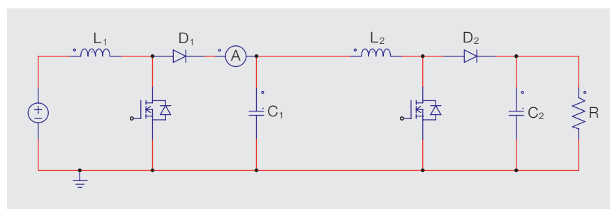
Figure 4 Hacheur élévateur de tension double boost en cascade.
