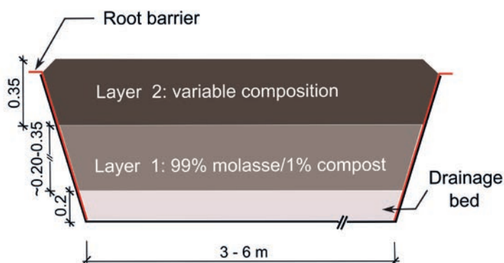
Schéma simplifié de la structure en trois horizons d'un technosol. croquis: C. Staudinger/OSL
